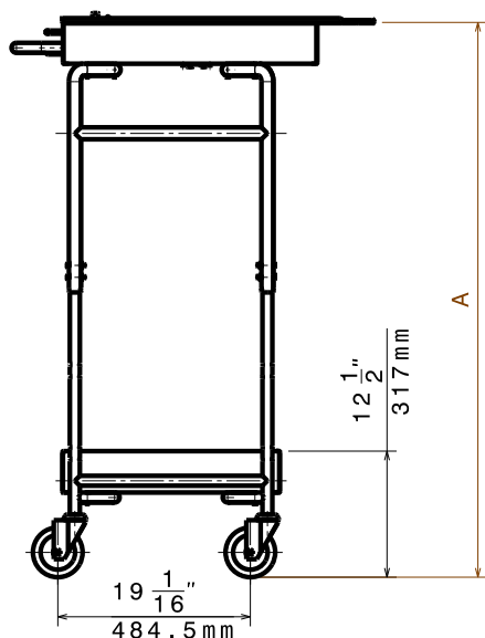
Zij aanzicht
