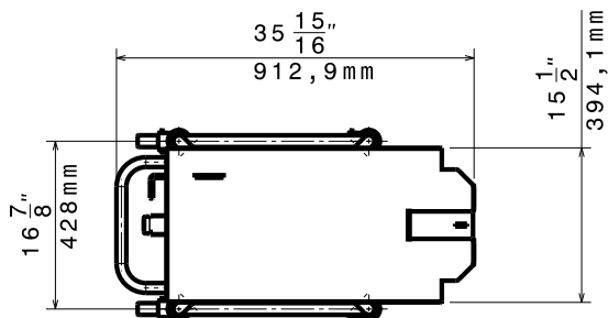
Boven aanzicht
